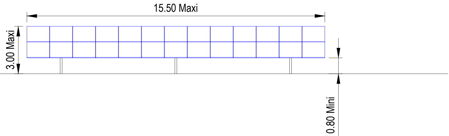
Vue de Face 2V13
