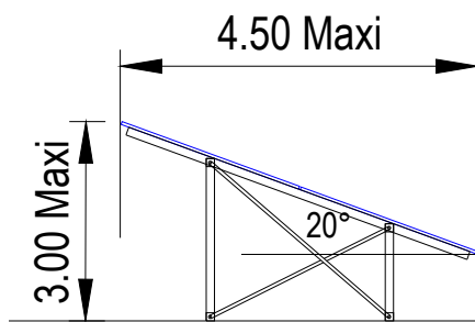
Vue de côté 2V13
